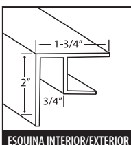
ESQUINA INTERIOR/EXTERIOR
